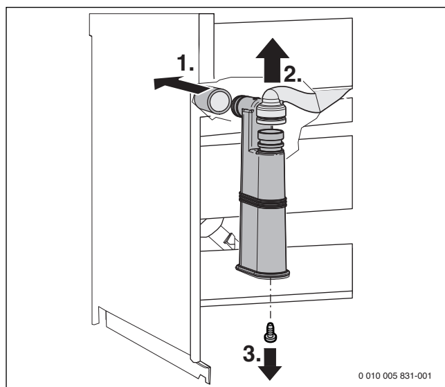
Рис. 54 Демонтаж конденсатного сифона
