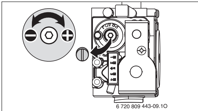
Рис. 42 Удаление пломбы с газовой арматуры
