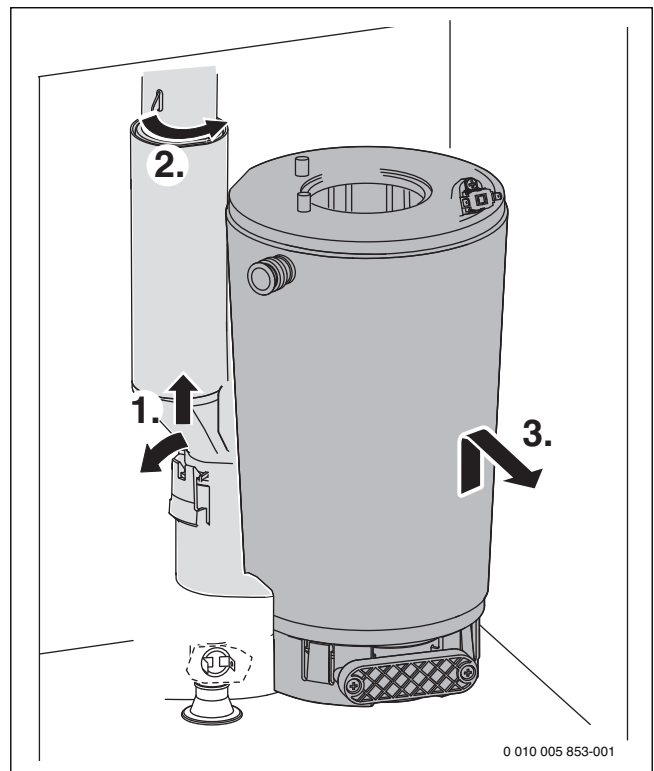
Рис. 66 Демонтаж теплообменника
