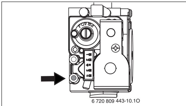
Рис. 43 Штуцер для измерения подаваемого давления газа
