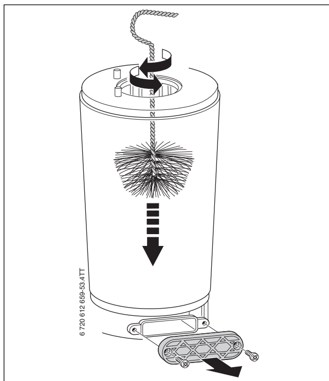
Рис. 51 Чистка теплообменника
