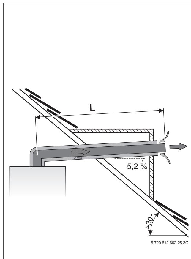
Рис. 13 Горизонтальный отвод дымовых газов по C_{13(x)}
