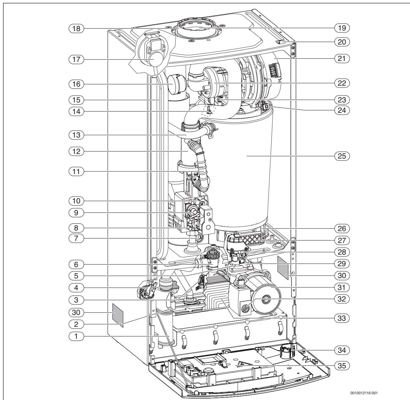
Рис. 3 Обзор котла
